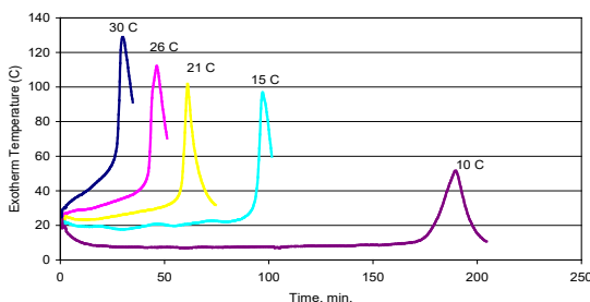
Typische Exotherm-Härtung bei MA550-30 (Masse 30 g) bei verschiedenen Umgebungstemperaturen 5
