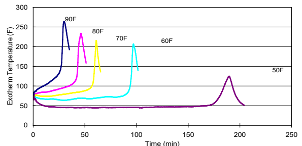
Typische Exotherm-Härtung bei MA550-30 (Masse 30 g) bei verschiedenen Umgebungstemperaturen 5
