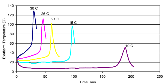
Curva exotérmica típica para el MA550 en masa de 30 g a varias temperaturas ambiente 5
