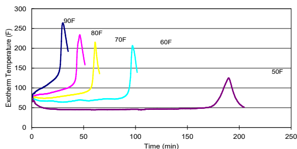
Curva exotérmica típica para el MA550 en masa de 30 g a varias temperaturas ambiente 5
