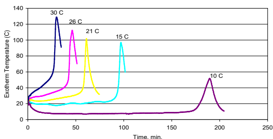
Courbe exothermique typique pour MA550 30 g en masse at Various Ambient Temperatures 5
