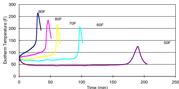
Courbe exothermique typique pour MA550 30 g en masse at Various Ambient Temperatures 5
