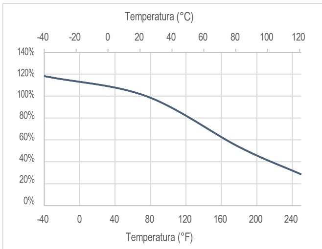
Retención de fuerza vs. temperatura (ASTM D1002 sobre AL6061)
