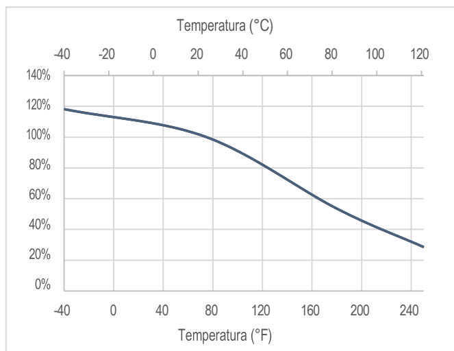
Mantenimento della resistenza vs Temperatura (ASTM D1002 su AL6061)
