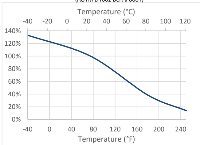
Temperaturabhängige Festigkeit (ASTM D1002 bei Al 6061)
