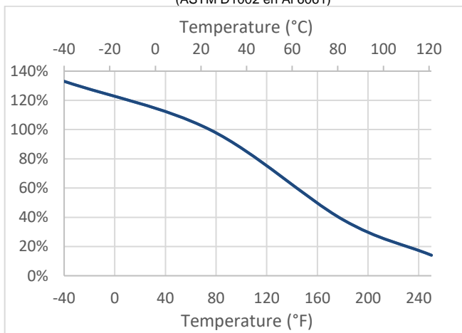
Retención de fuerza vs. temperatura (ASTM D1002 en Al 6061)
