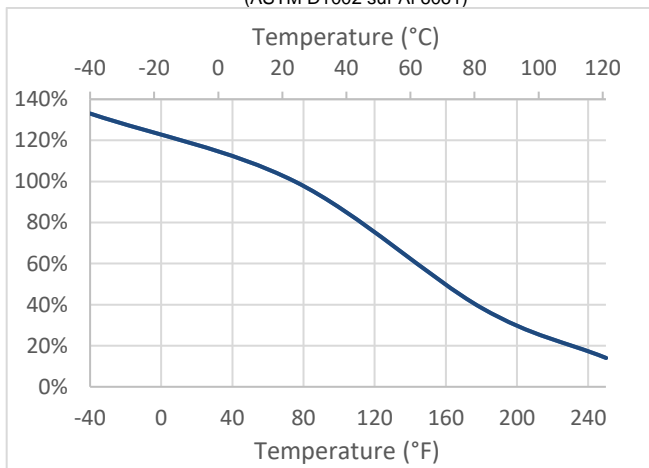
Degré de résistance en fonction de la température (ASTM D1002 sur Al 6061)
