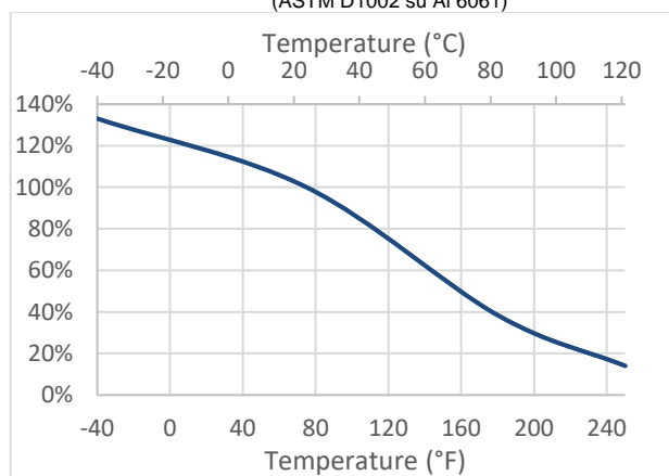
Mantenimento della resistenza vs temperatura (ASTM D1002 su AI 6061)
