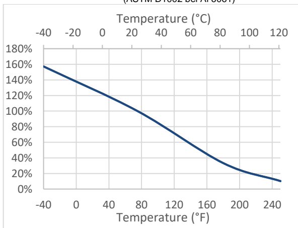
Temperaturabhängige Festigkeit (ASTM D1002 bei Al 6061)
