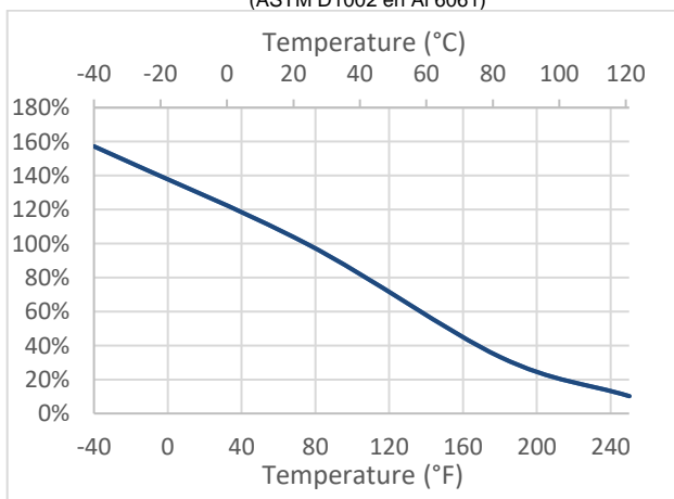
Retención de fuerza vs. temperatura (ASTM D1002 en Al 6061)
