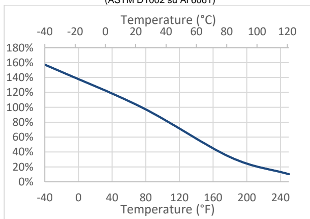
Mantenimento della resistenza vs temperatura (ASTM D1002 su Al 6061)
