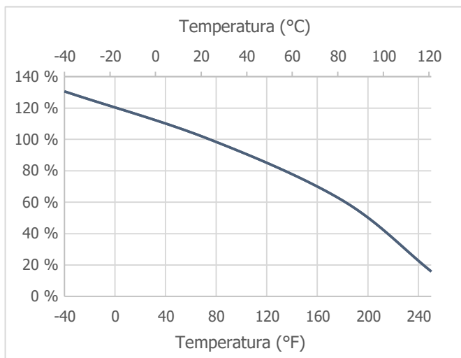
Retención de fuerza vs. temperatura (ASTM D1002 en AI 6061)
