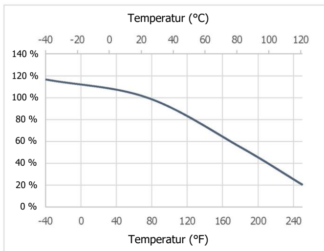
Temperaturabhängige Festigkeit (ASTM D1002 bei AI 6061)
