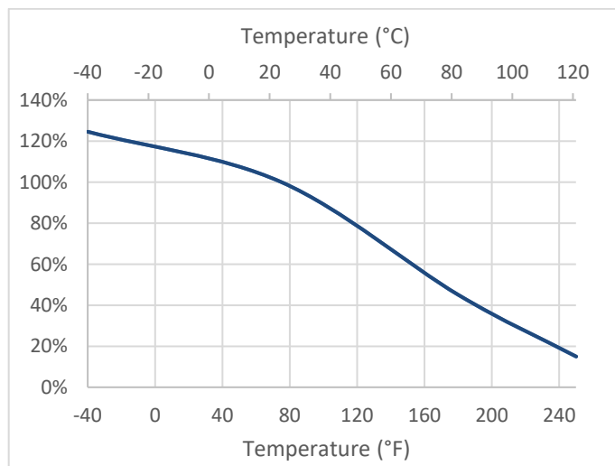
Retención de fuerza vs. temperatura (ASTM D1002 en AI 6061)
