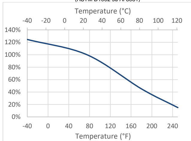
Mantenimento della resistenza vs temperatura (ASTM D1002 su AI 6061)
