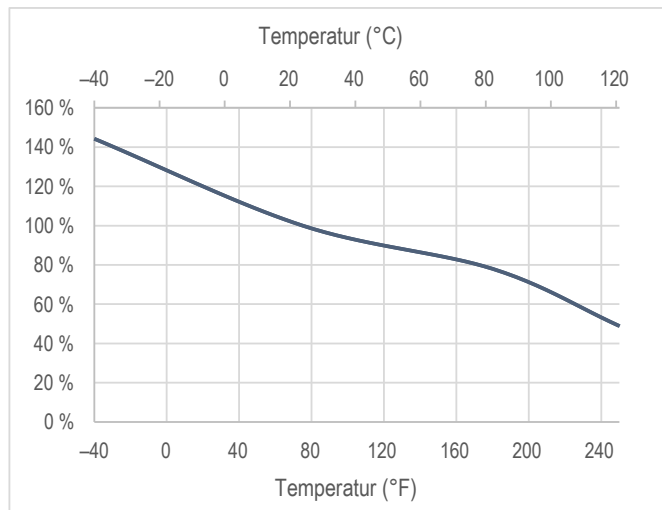
Temperaturabhängige Festigkeit (ASTM D1002 bei Al 6061)
